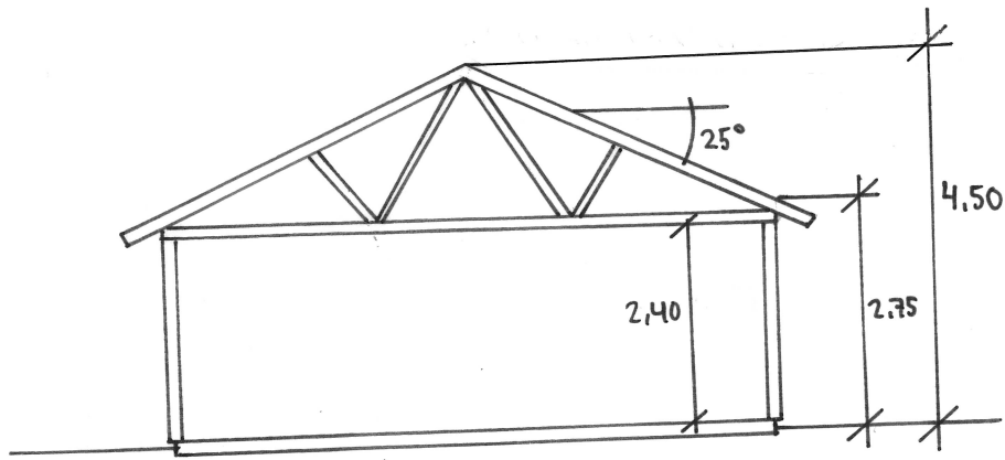
Sektion A-A
